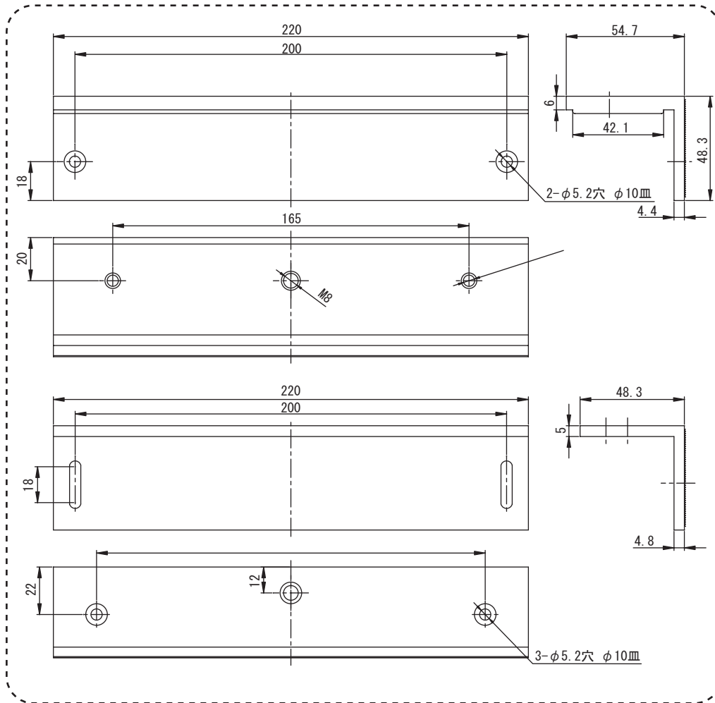
【Zブラケット】
