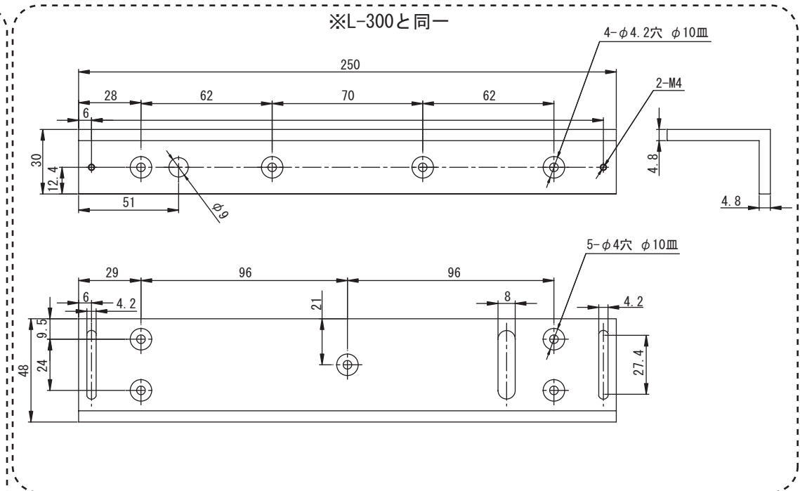
【Lブラケット】
