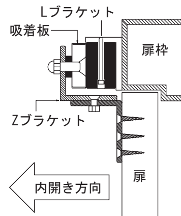
Zブラケット
